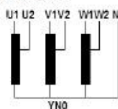
Fig.2: Elektrisch Schema
